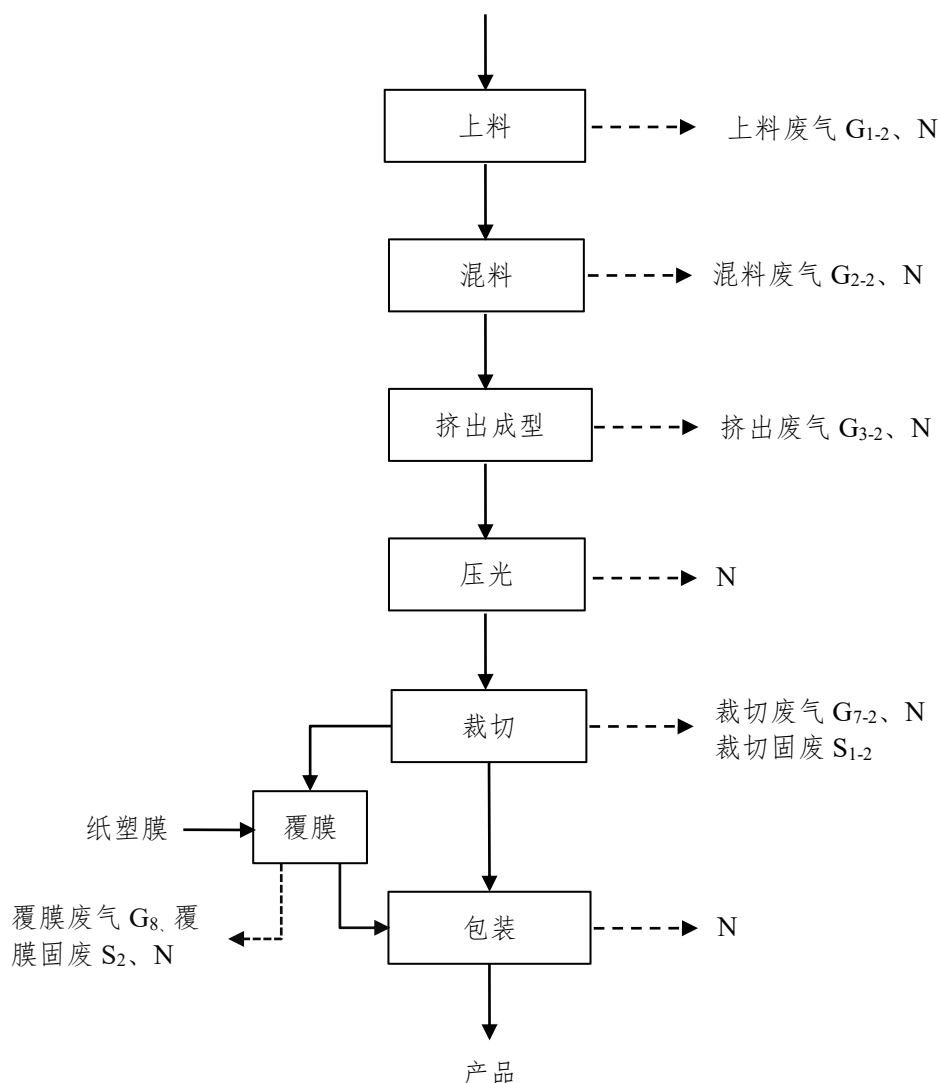
图 2-2 挤出板生产流程及产排污环节图
