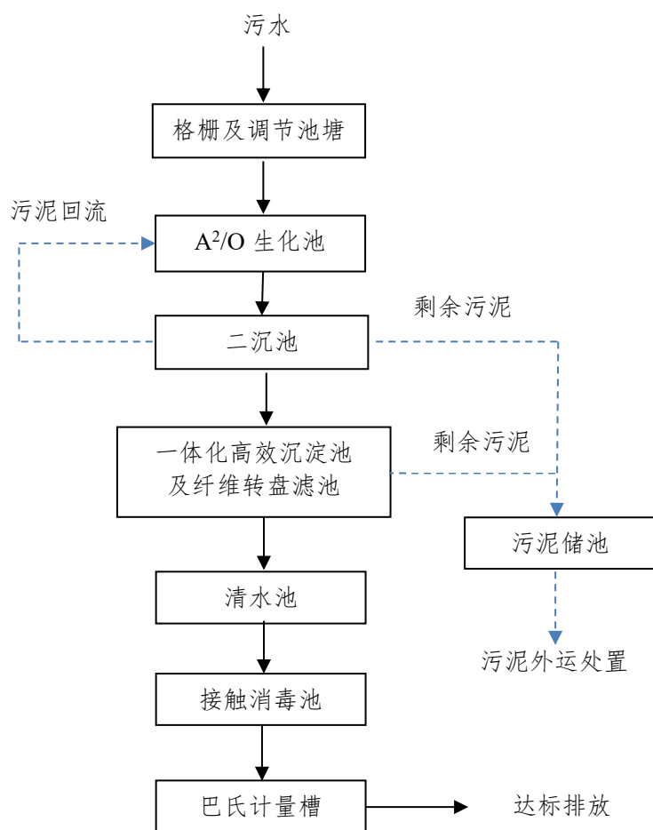
图 4-2 蔡桥镇污水处理厂处理工艺
