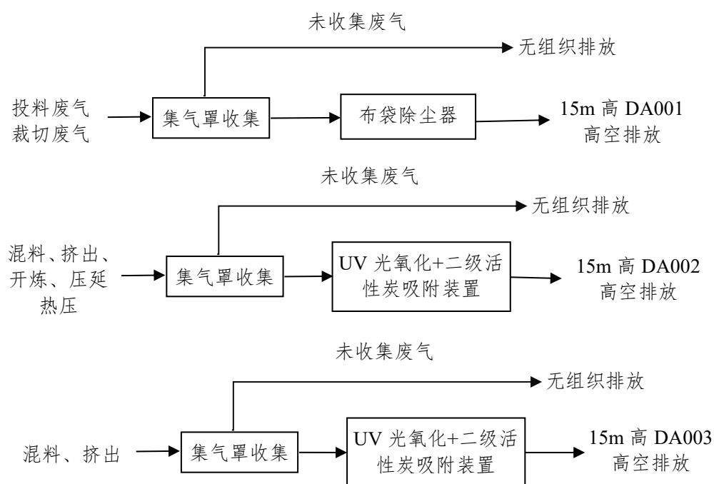
图 4-1 建设项目废气处理工艺流程图
