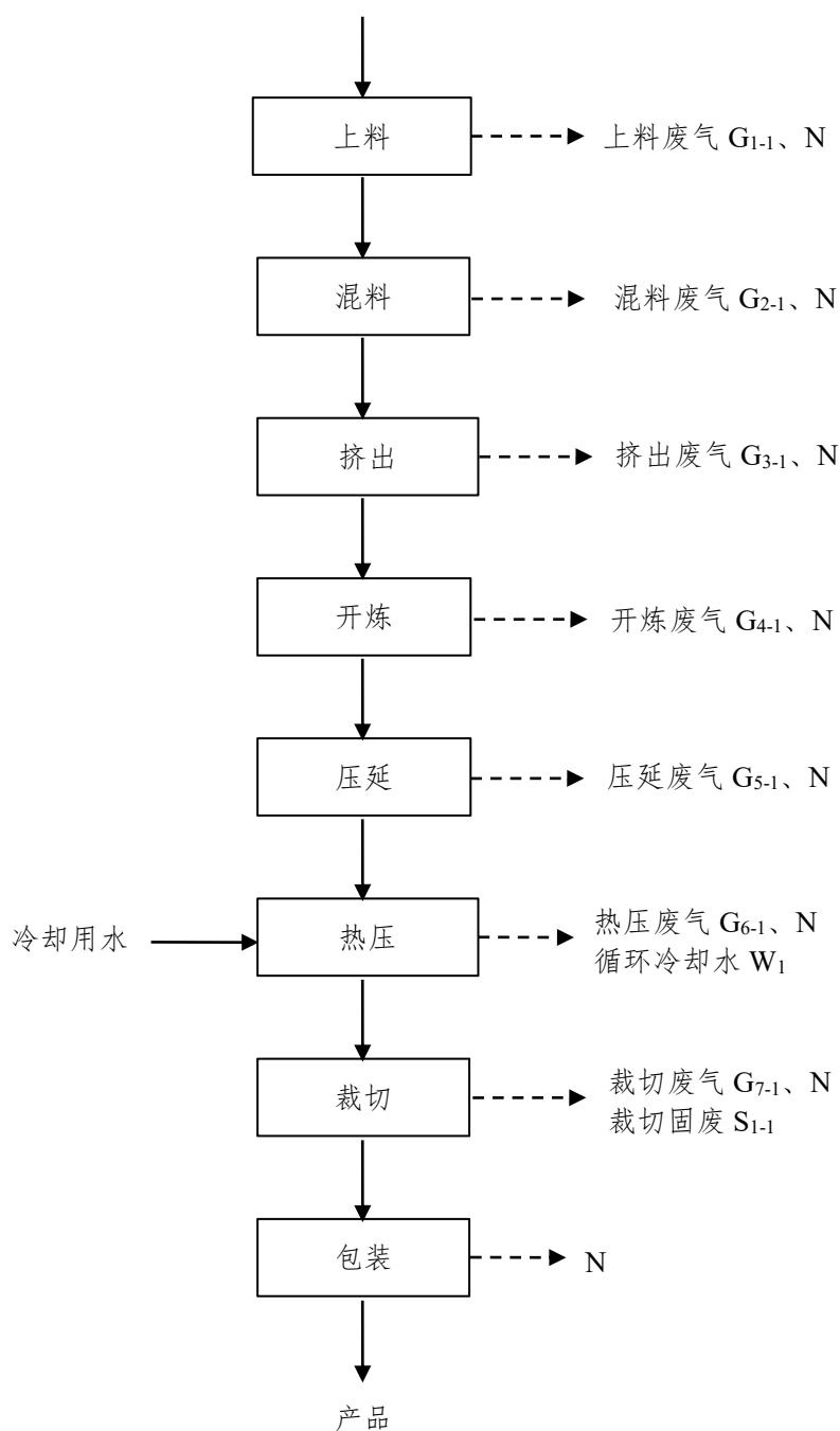
图 2-1 层压板生产流程及产排污环节图
