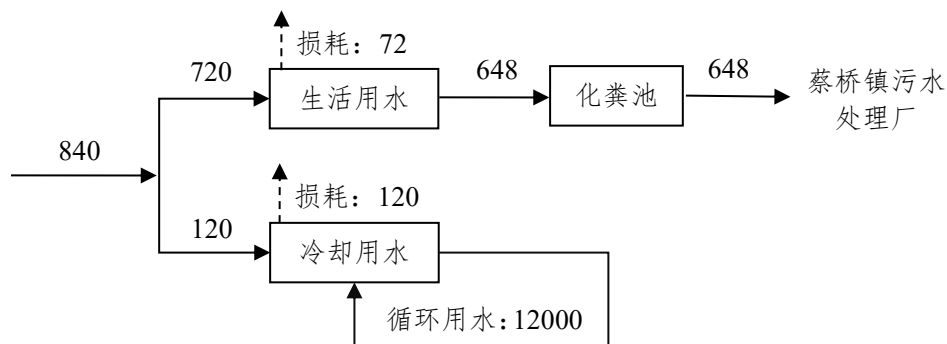
图 2-2 建设项目水平衡图 (t/a)
