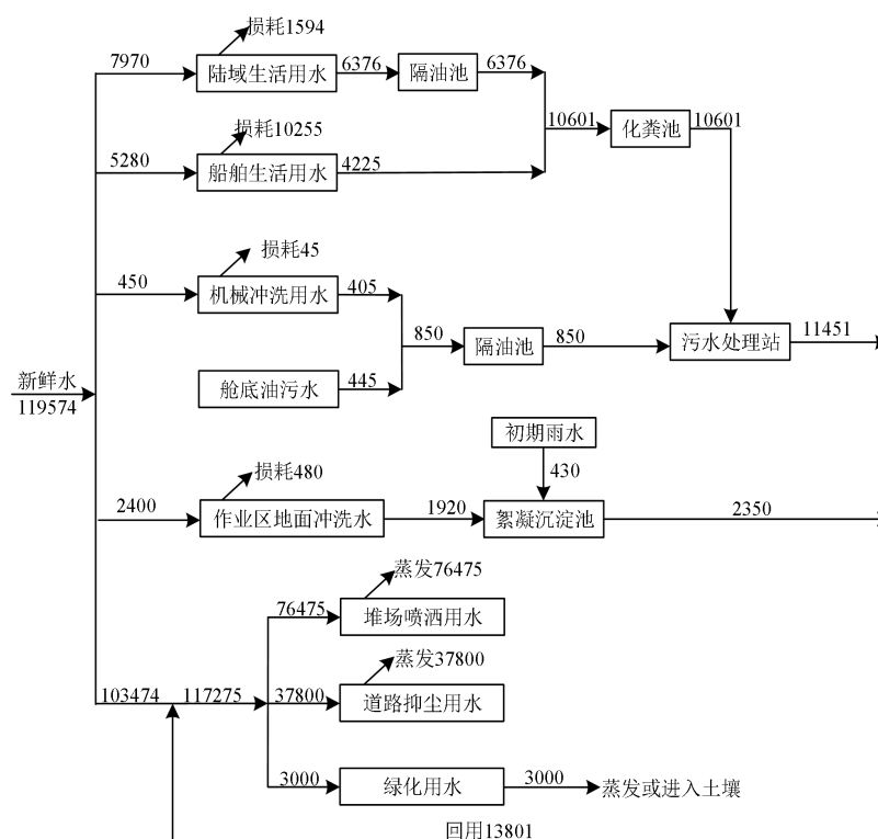
图 2-5 现有项目水平衡图 单位 t/a
