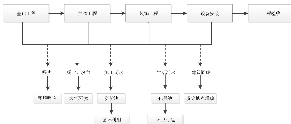
图 4-1 施工期工程工艺流程图
