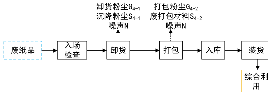
图 2-5 废纸品处理的工艺流程及产污节点图
