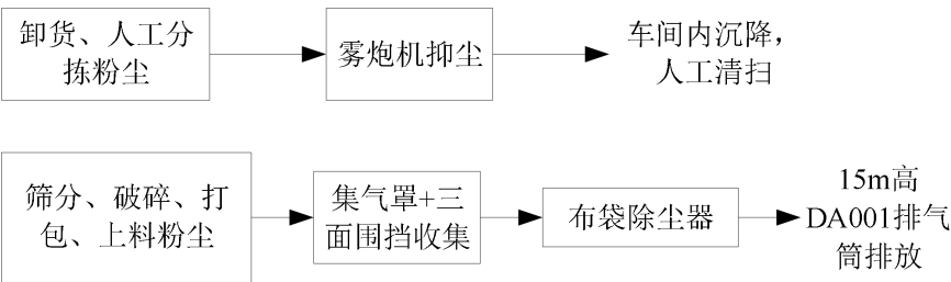
图 4-1 废气处理示意图
