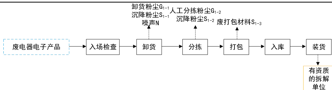
图 2-2 废电器电子产品处理的工艺流程及产污节点图
